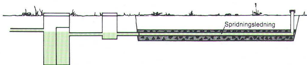
Slamavskiljare Fördelningsbrunn
